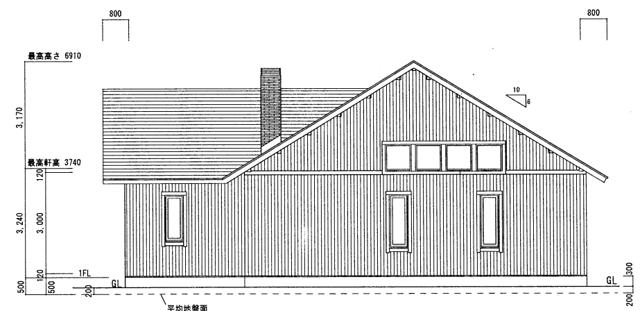
南側 立面図 S=1:100
