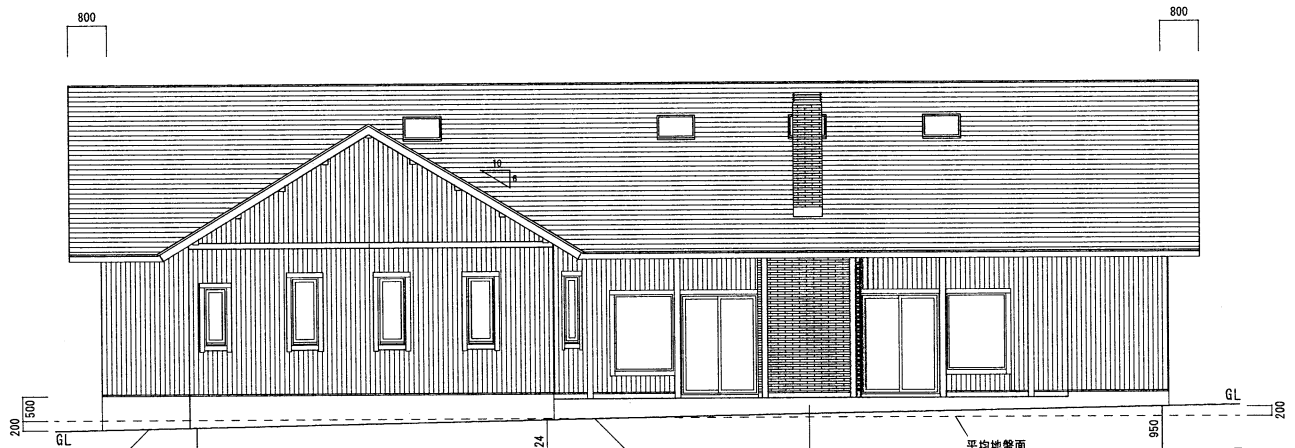
西側 立面図 S=1:100
